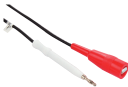
耐压输出线 - 鳄鱼夹 (12 kV)
